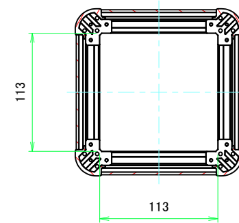
C-C (1:3.5)
